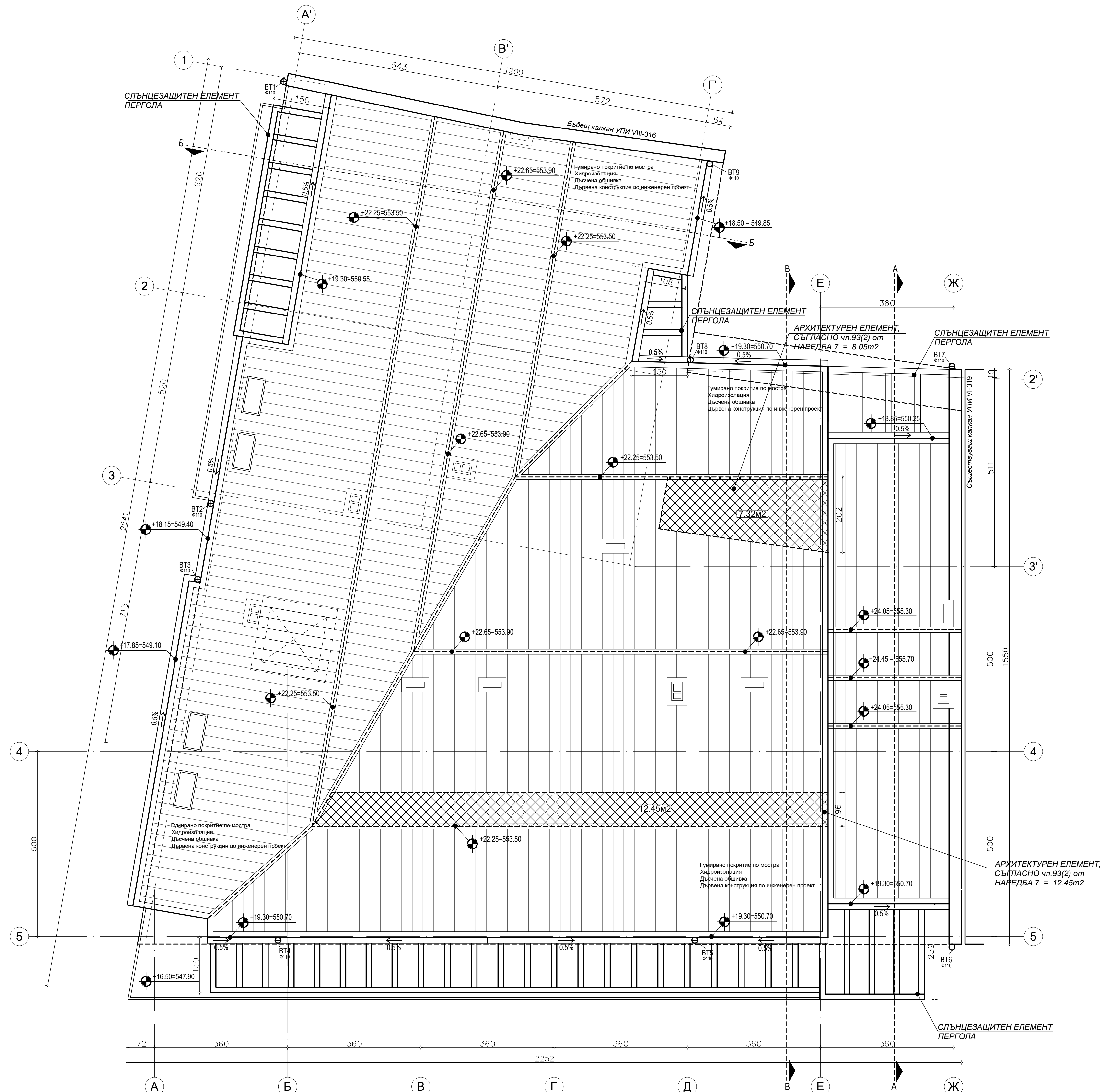
ПЛАН ПОКРИВ М 1:50
