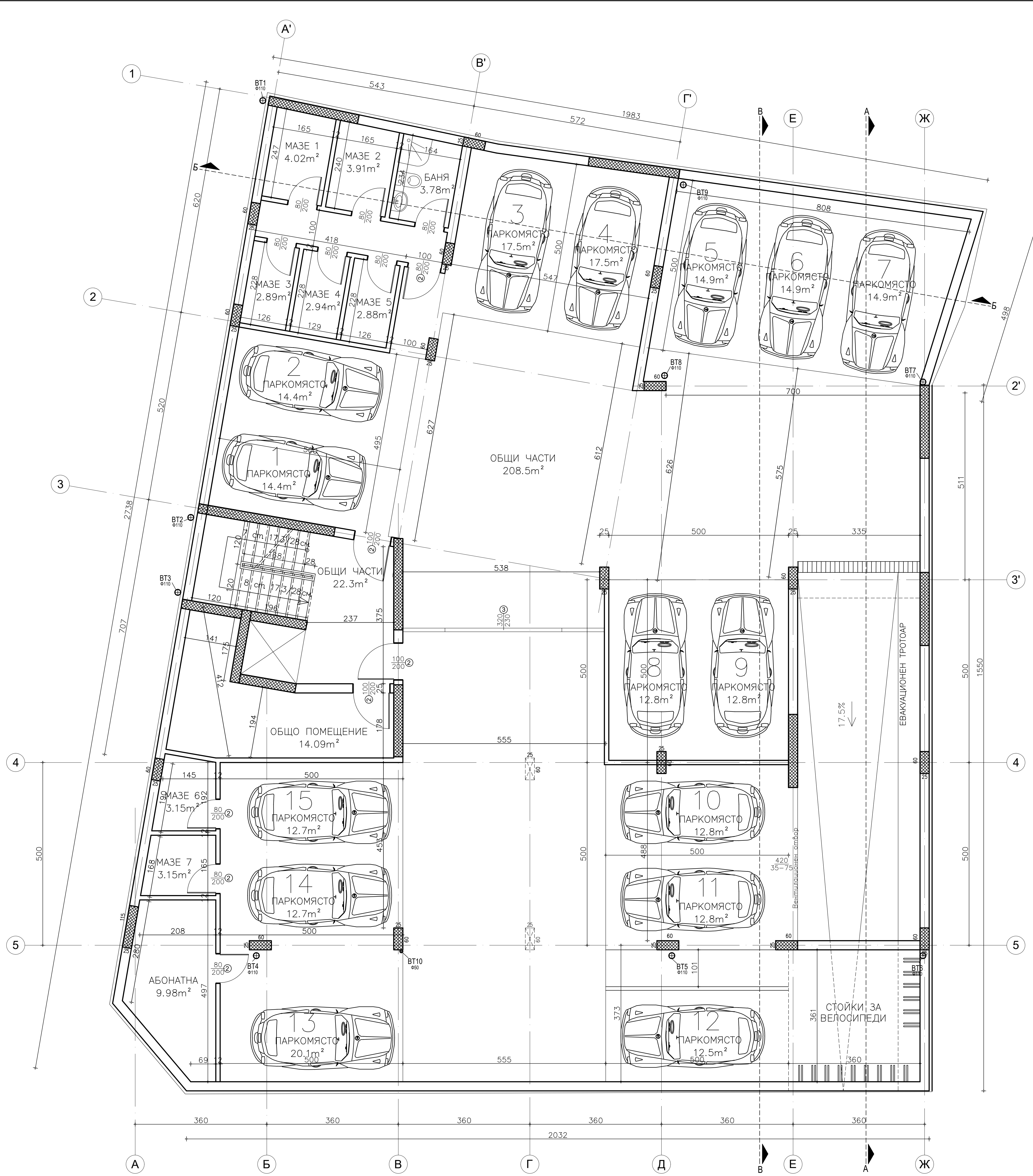
РАЗПРЕДЕЛЕНИЕ НА ПОДЗЕМЕН ГАРАЖ - НИВО -2.60 - 528.80 = 451.83м 2
