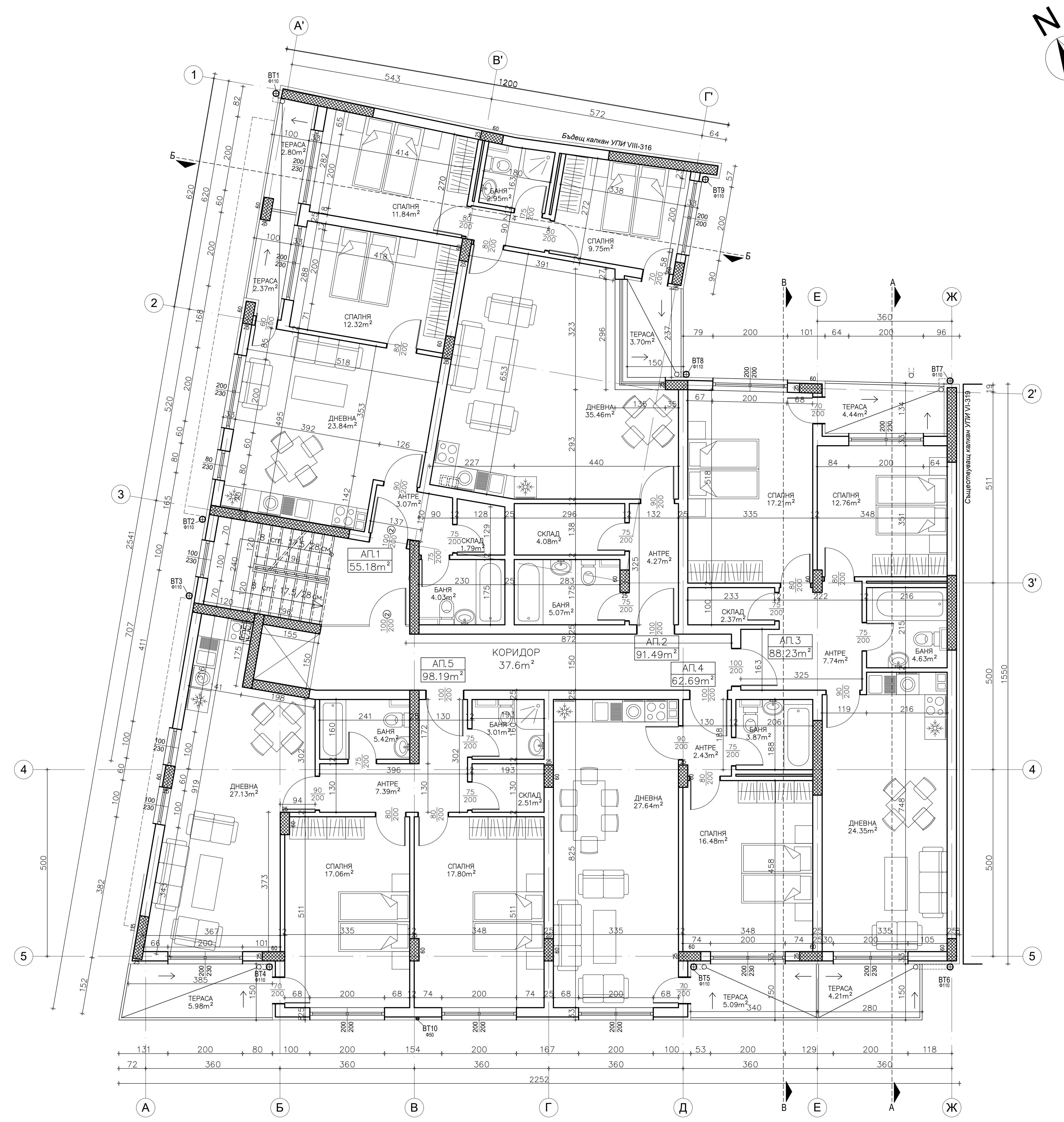
РАЗПРЕДЕЛЕНИЕ НА ПЪРВИ ЕТАЖ - НИВО +2.50 - 533.90 = 433.74m2
