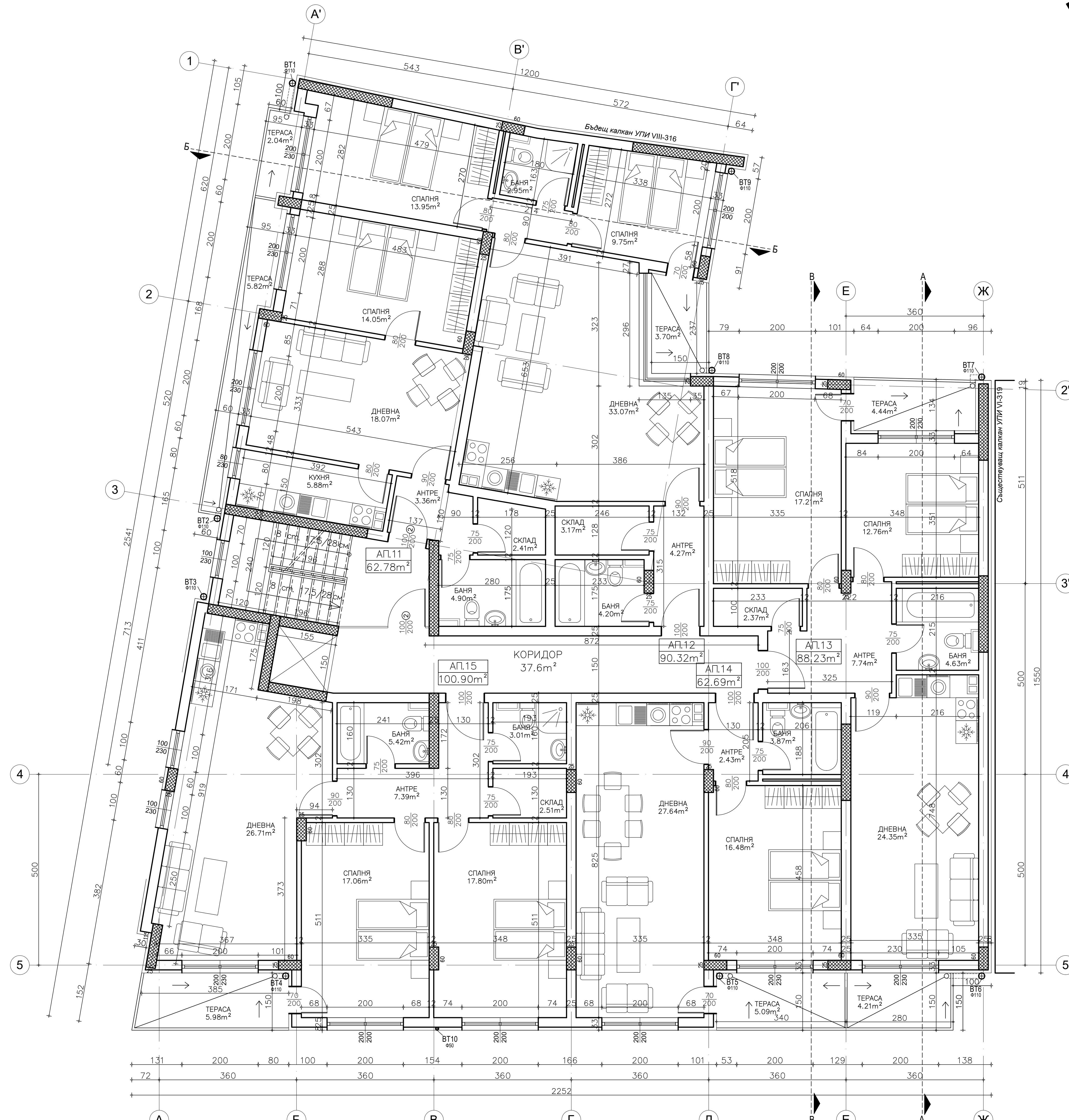
РАЗПРЕДЕЛЕНИЕ НА ТРЕТИ ЕТАЖ - НИВО +8.10 - 539.50 = 442.87m2
